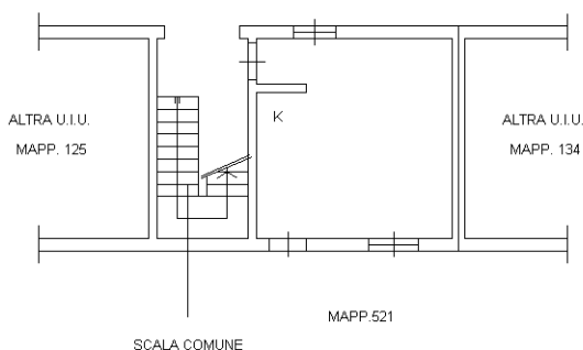
PIANTA PIANO TERRA H=300
