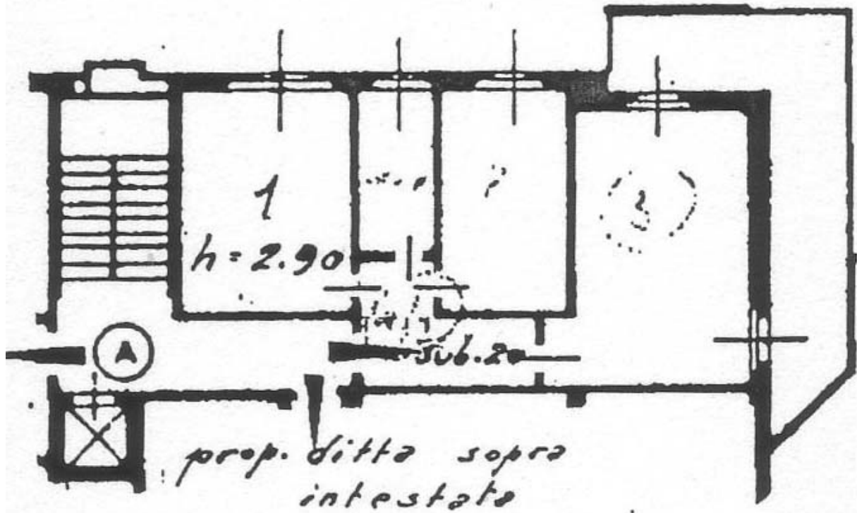
Planimetria appartamento - piano quarto
