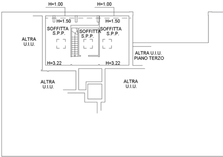
PIANO QUARTO (SOTTOTETTO)
