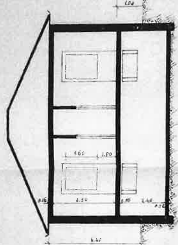
Sezione trasversale
