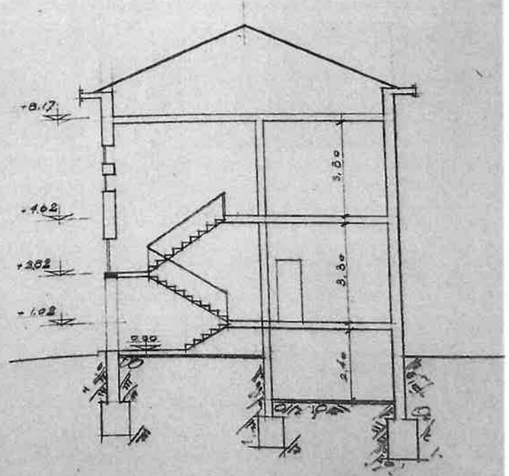
SEZIONE A-B
