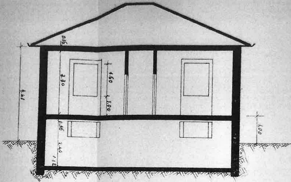
sezione trasversale
