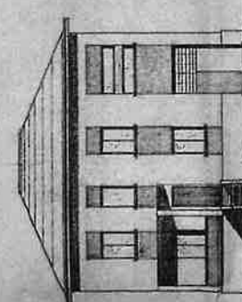
PROSPETTO OVEST
