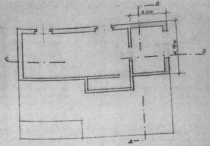
PIANTA SEMINTERRATO
