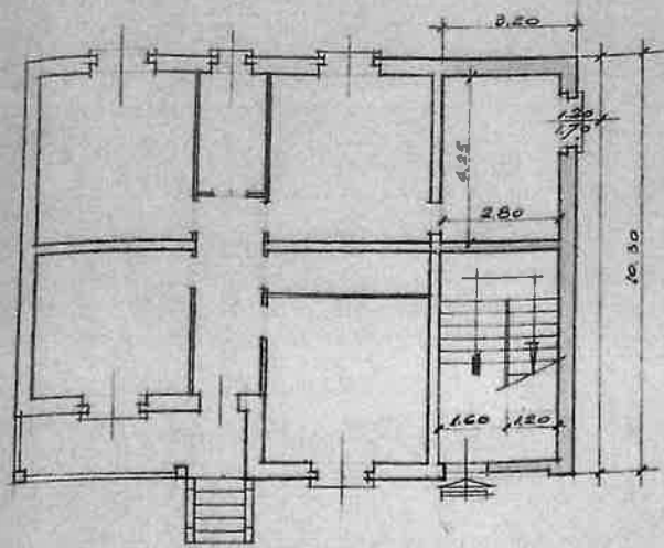
PIANTA DIAMO TERRA
