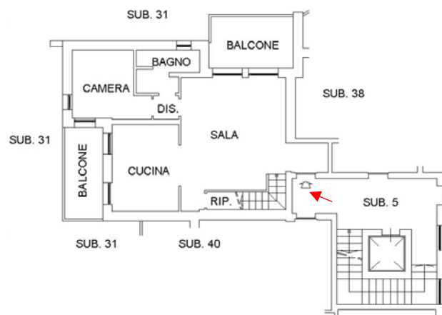
PIANO SECONDO ABITAZIONE H=2,70
